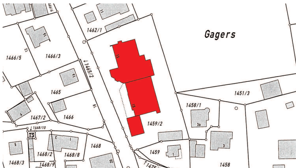
LAGEPLAN BADSTRASSE 13 - 15
